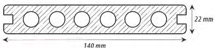
Przekrój
